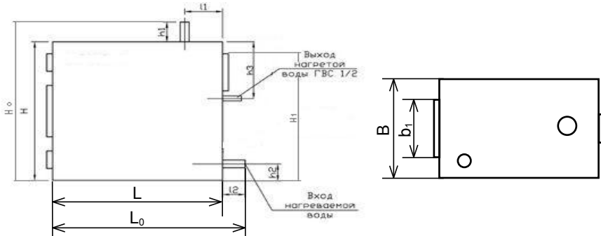
Рис. 1 — Чертеж Изделия
